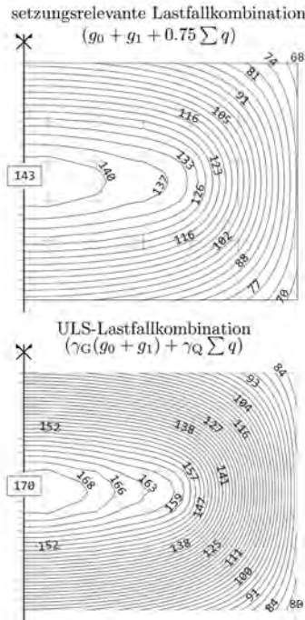
Bild 46. Setzungsmulde für die setzungsrelevante Lastfallkombination und implizit vergrößerte Setzungsmulde im gebetteten 3D-Gesamtmodell durch die ULS-Lastfallkombination und Teilsicherheitsbeiwerte für äußere Lasten im ULS
